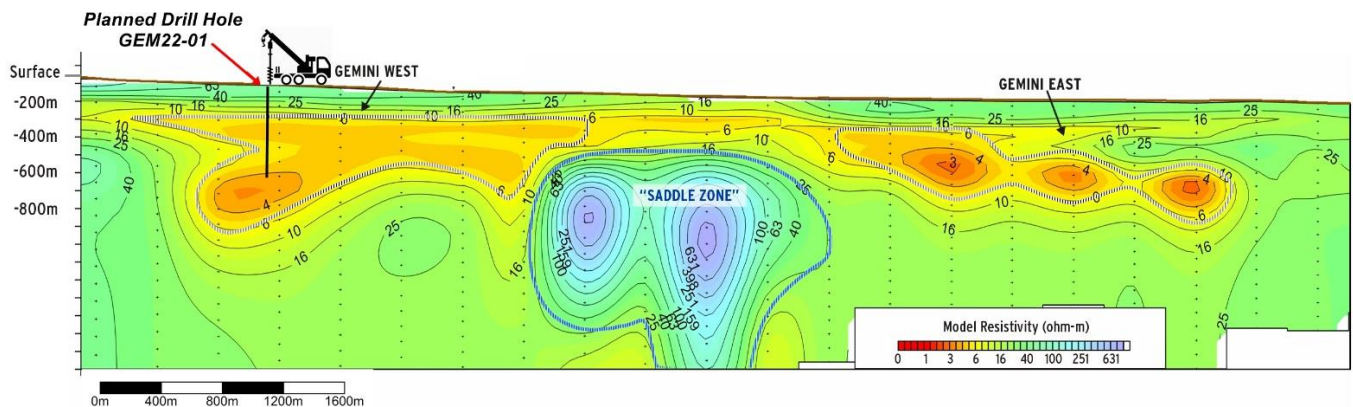
Gemini Lithium Project Time-Domain EM Section
